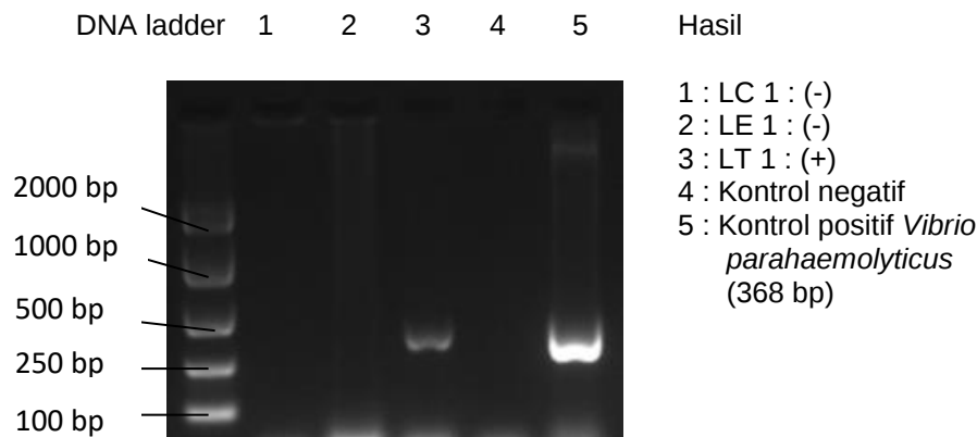
Gambar 1. Visualisasi elektroforesis DNA dengan metode Boilling Lysis Buffer untuk ulangan 1
