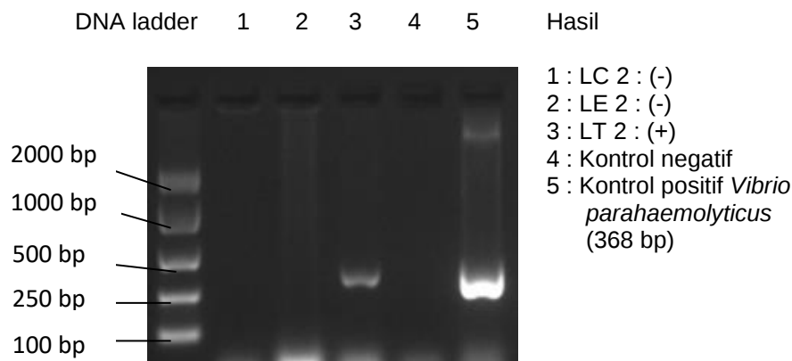
Gambar 2. Visualisasi elektroforesis DNA dengan metode Boilling Lysis Buffer untuk ulangan 2
