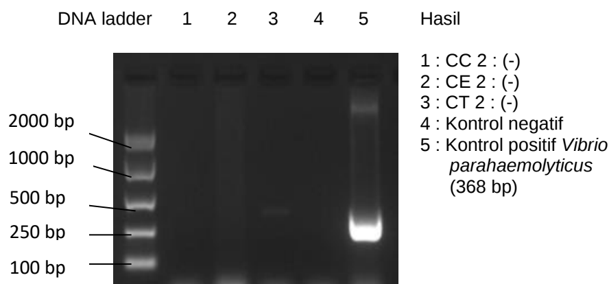
Gambar 4. Visualisasi elektroforesis DNA dengan metode Chloroform untuk ulangan 2
