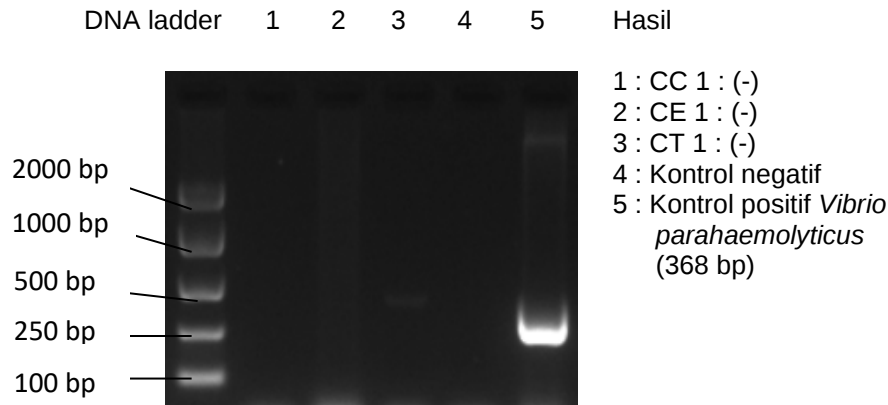
Gambar 3. Visualisasi elektroforesis DNA dengan metode Chloroform untuk ulangan 1
